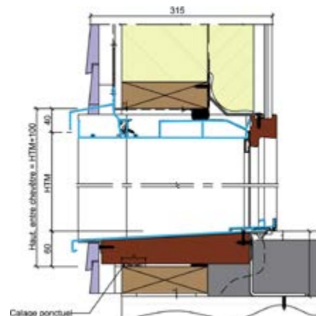
COUPE VERTICALE
