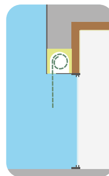
Coffre linteau enroulement intérieur
