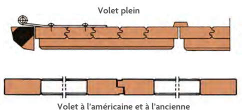
Coupes, volets pleins et persiennés
