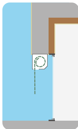
Pose en tunnel enroulement intérieur
