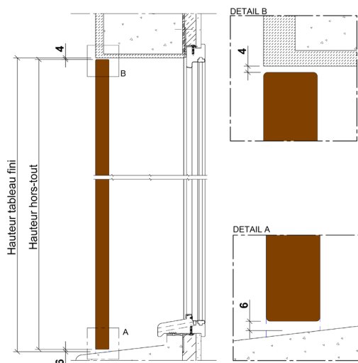
Coupe verticale avec détails
