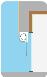
Pose en tunnel enroulement extérieur
