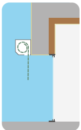
Pose en applique enroulement extérieur
