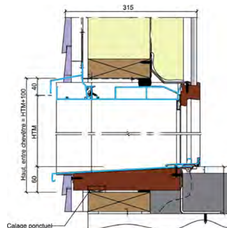
COUPE VERTICALE
