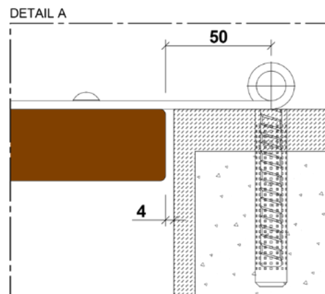
Position du gond
