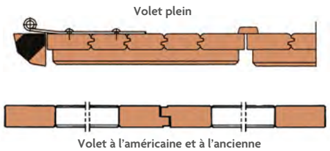
Coupes, volets pleins et persiennés
