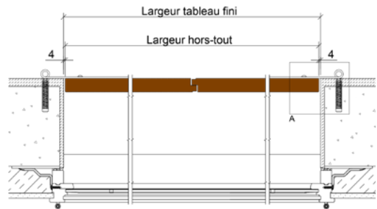
Coupe horizontale
