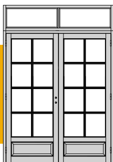
Imposte vitrée avec meneau sur porte 2 vantaux
