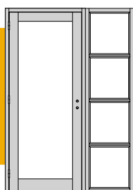
Fixe latéral avec traverses intermédiaires
